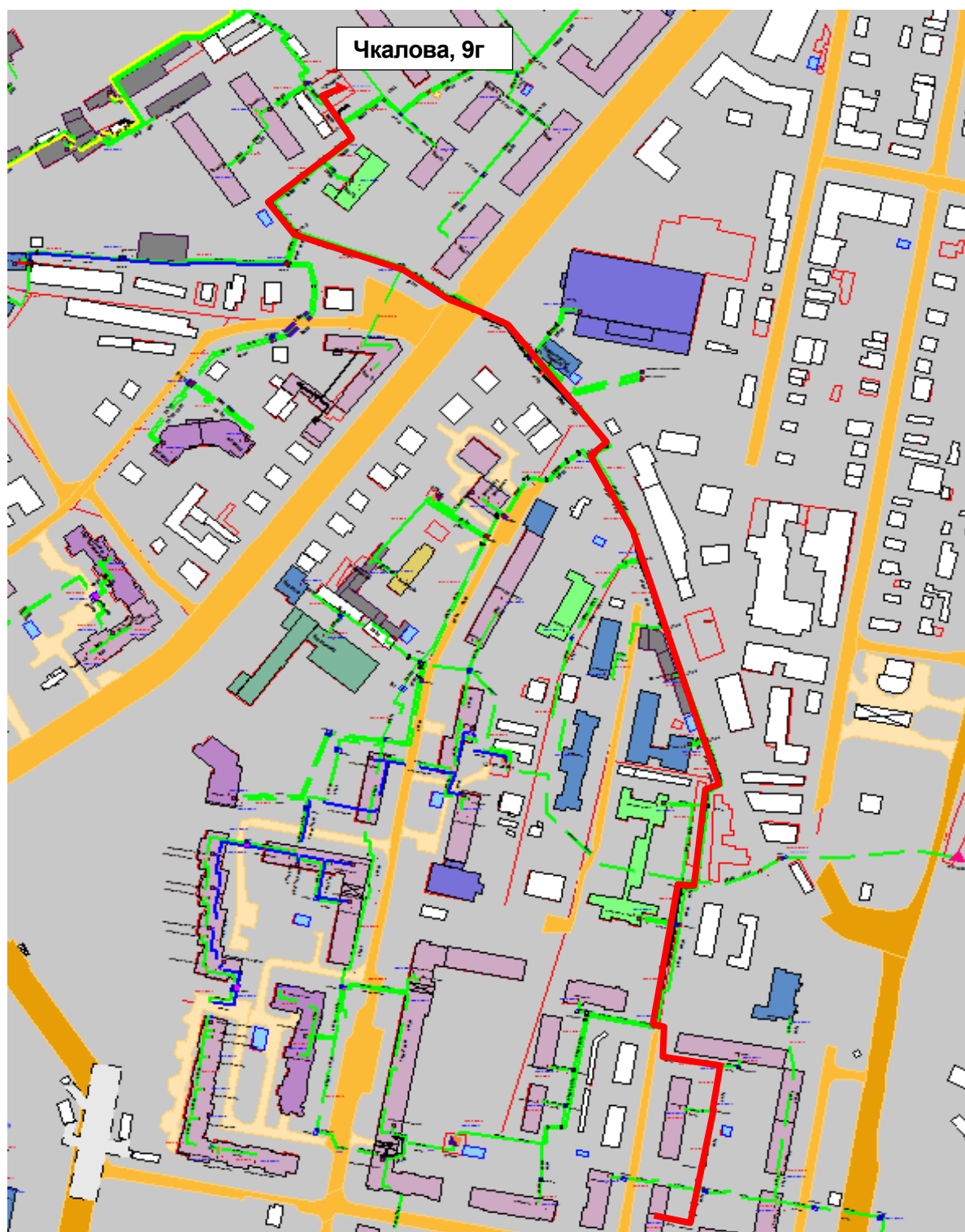
Рисунок 1.117 – Результат гидравлического расчета - расчетный путь теплоносителя от котельной Чкалова, 9г до ПТ-Вольск,8
