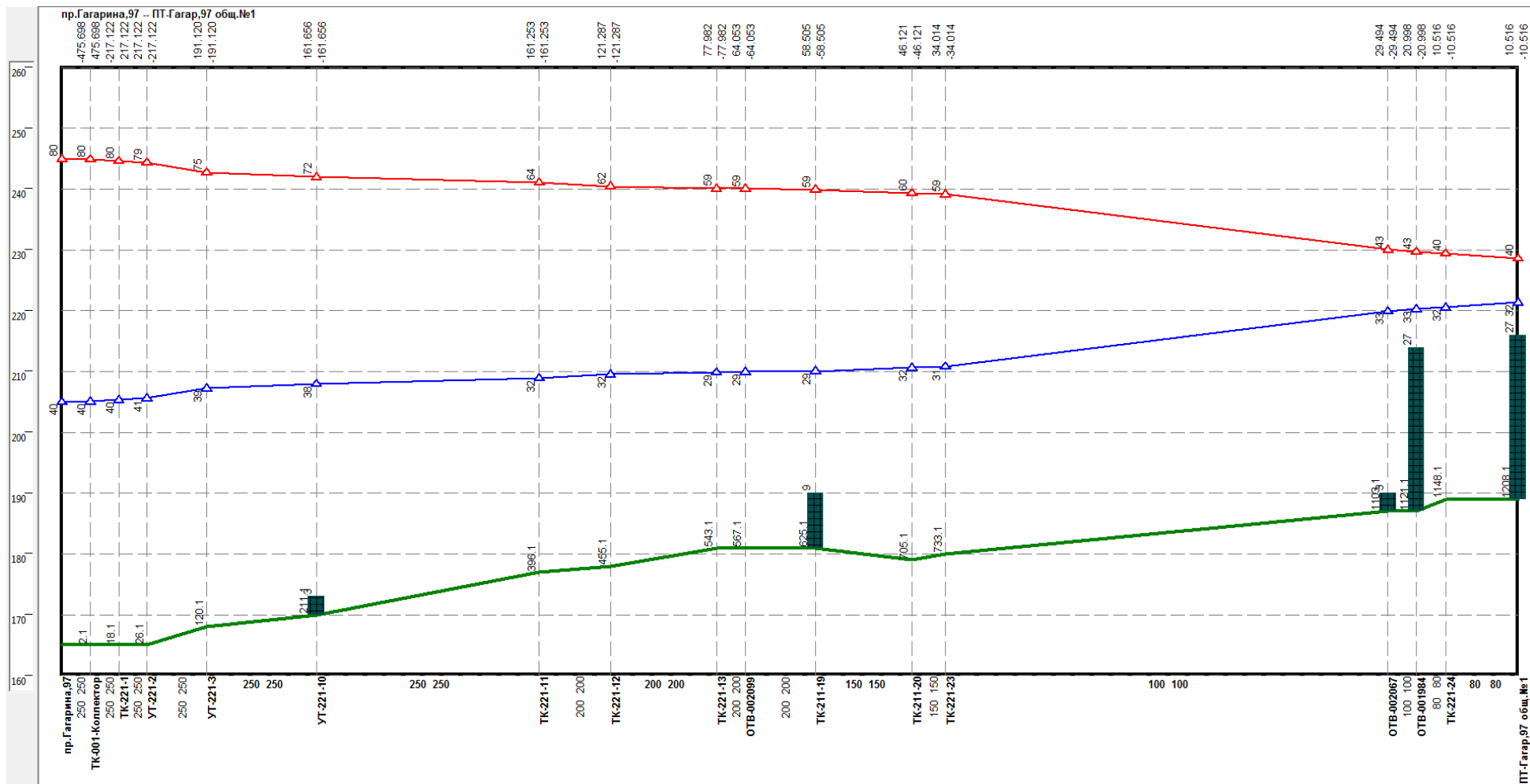
Рисунок 1.34 –Результат гидравлического расчета - график гидравлических режимов по пути теплоносителя от котельной пр. Гагарина, 97 до ПТ-Гагар,97 общ.№1
