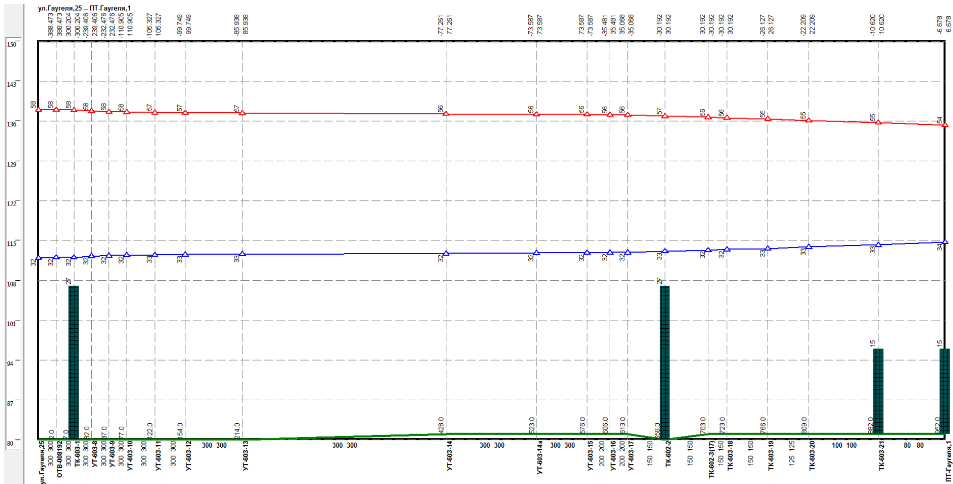
Рисунок 1.78 –Результат гидравлического расчета - график гидравлических режимов по пути теплоносителя от котельной ул. Гаугеля, 25 до ПТ-Гаугеля, 1
