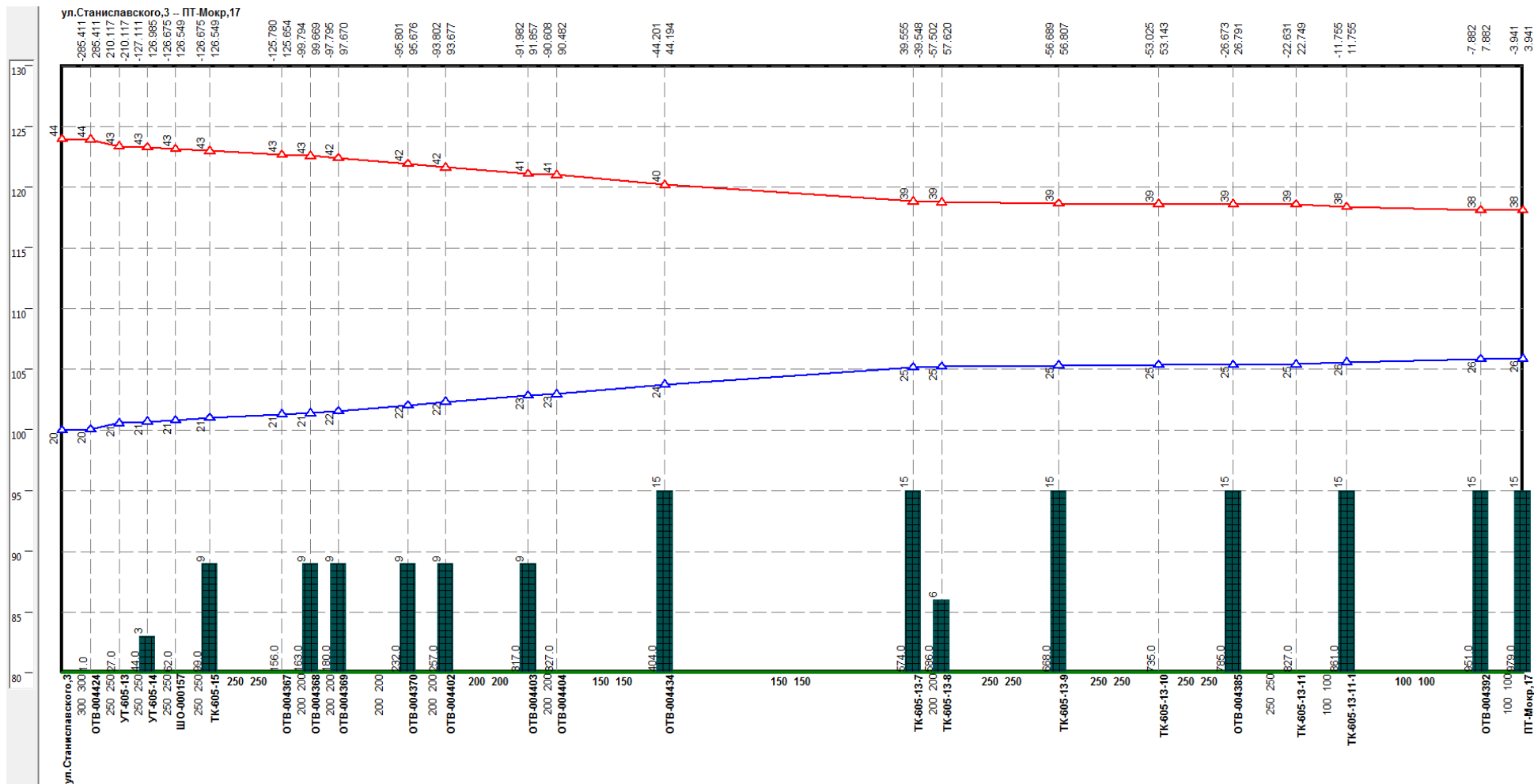
Рисунок 1.48 –Результат гидравлического расчета - график гидравлических режимов по пути теплоносителя от котельной Станиславского, 3 до ПТ-Мокр, 17
