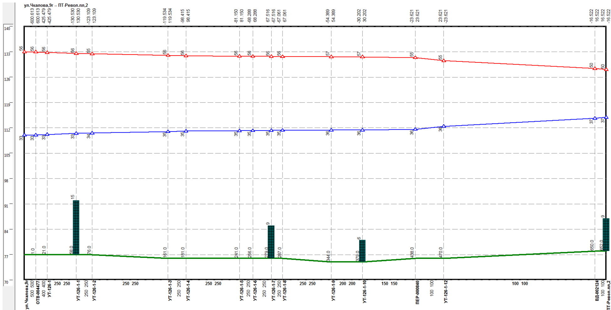
Рисунок 1.116 –Результат гидравлического расчета - график гидравлических режимов по пути теплоносителя от котельной Чкалова, 9д до ПТ-Революц.пл.2
