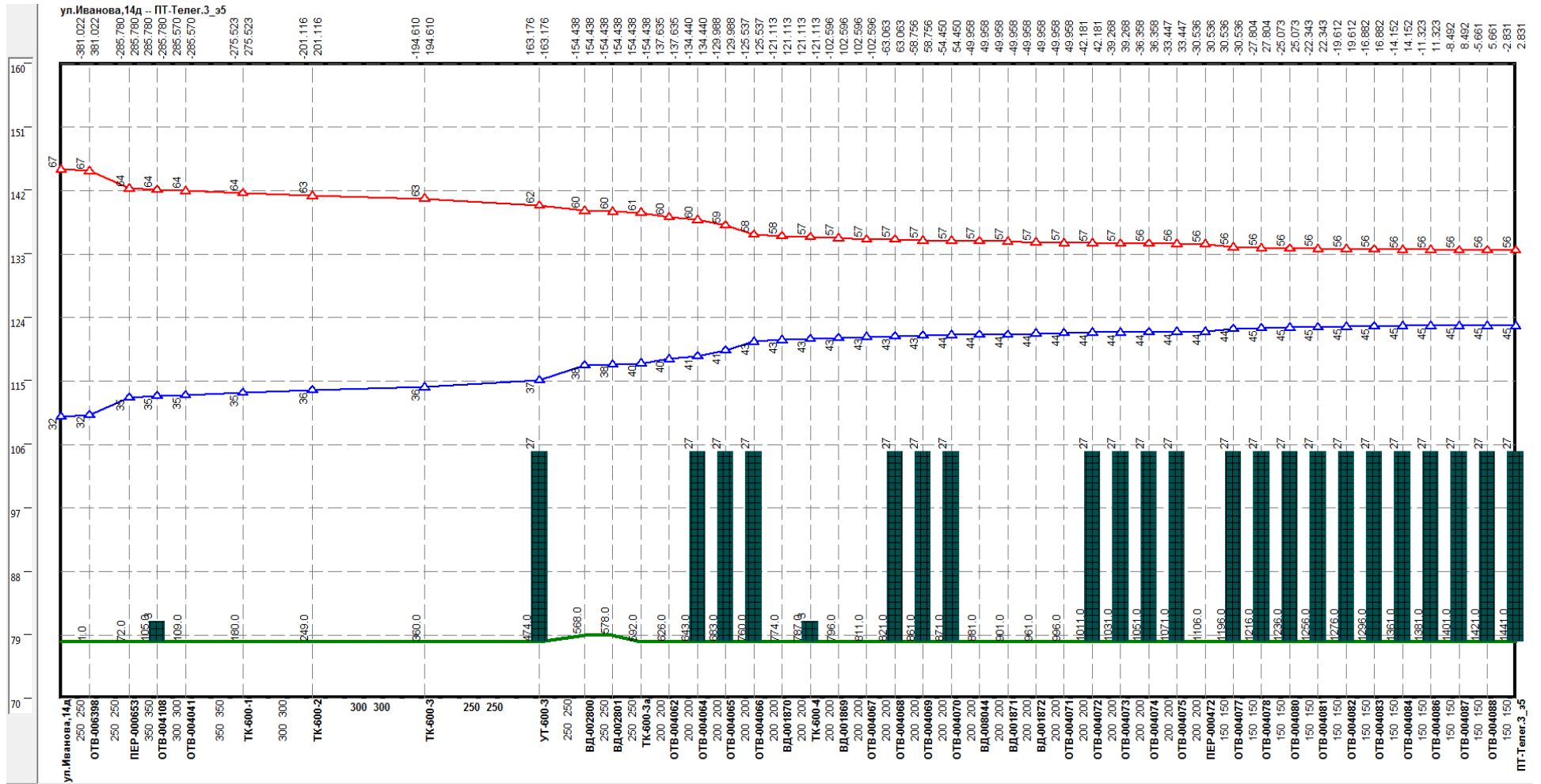
Рисунок 1.82 –Результат гидравлического расчета - график гидравлических режимов по пути теплоносителя от котельной ул. Иванова, 14б до ПТ-Телер.3_э5
