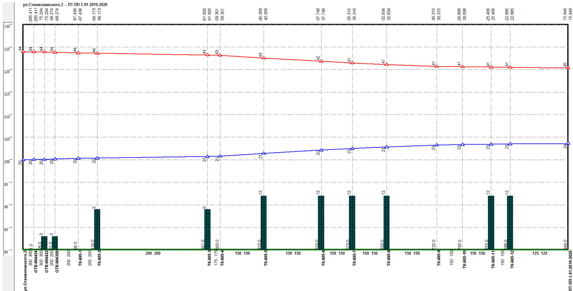
Рисунок 1.46 –Результат гидравлического расчета - график гидравлических режимов по пути теплоносителя от котельной Станиславского, 3 до ПТ-ПП-1.91-2019-2020
