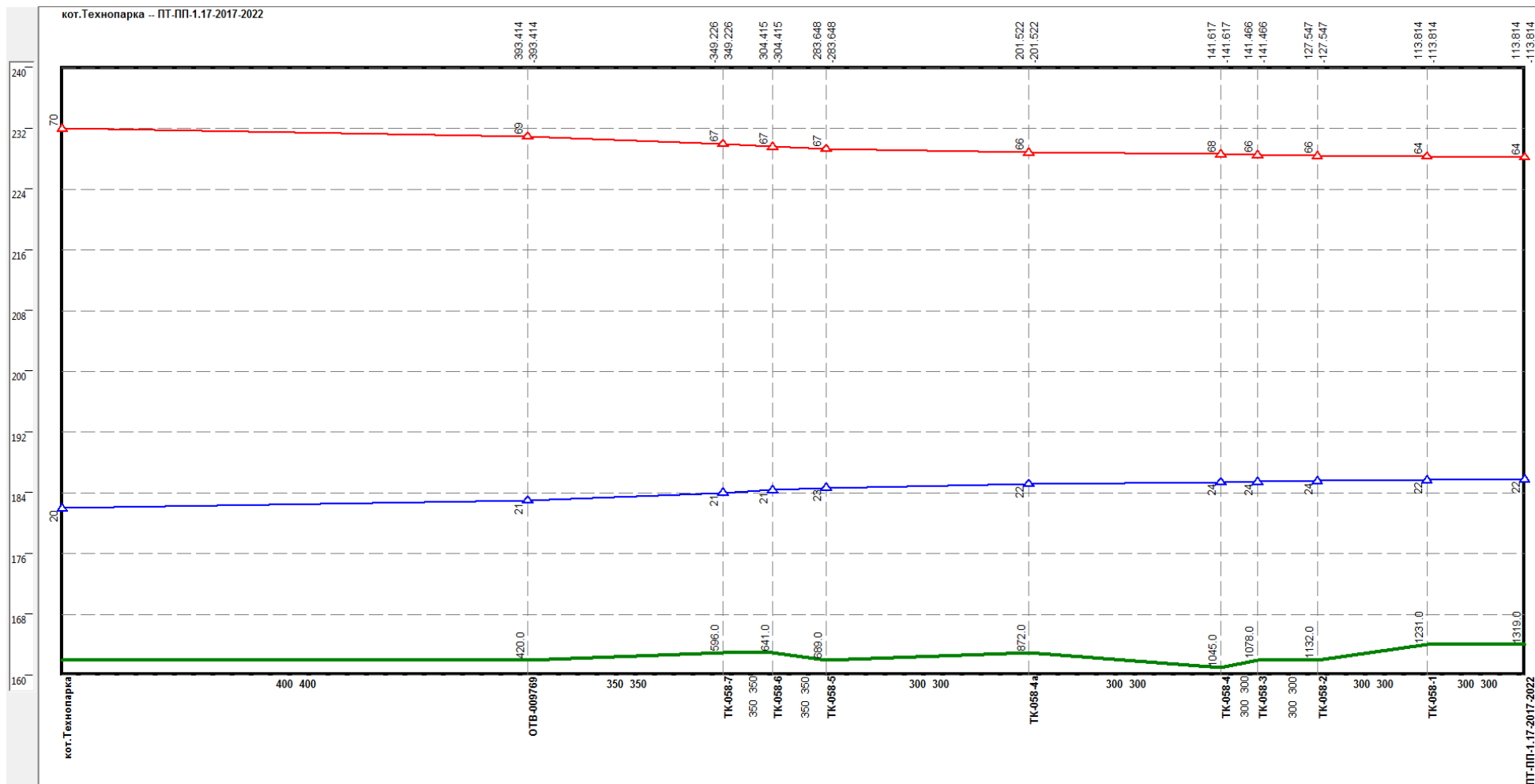
Рисунок 1.70 –Результат гидравлического расчета - график гидравлических режимов по пути теплоносителя от котельной «Технопарк» до ПТ-ПП-1.17-2017-2022
