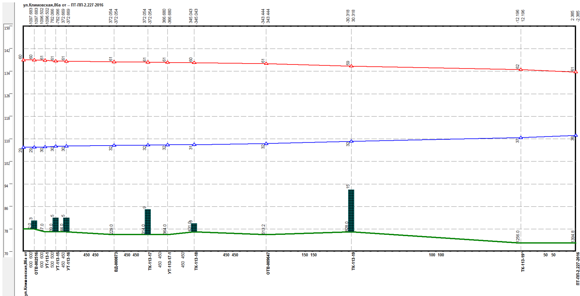
Рисунок 1.42 –Результат гидравлического расчета - график гидравлических режимов по пути теплоносителя от котельной Климовская, 86а до ПТ-ПП-2.227-2016
