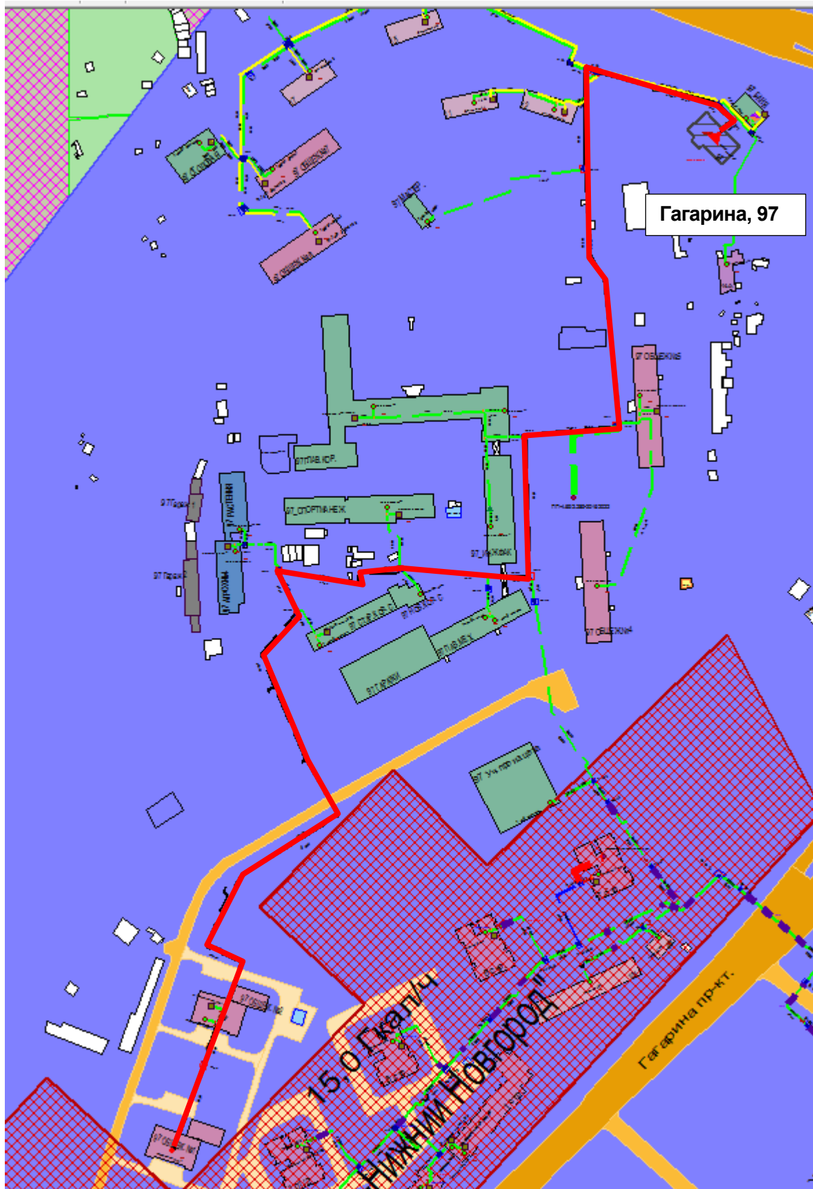
Рисунок 1.33 – Результат гидравлического расчета - расчетный путь теплоносителя от котельной пр. Гагарина, 97 до ПТ-Гагарин,97 общ.№1
