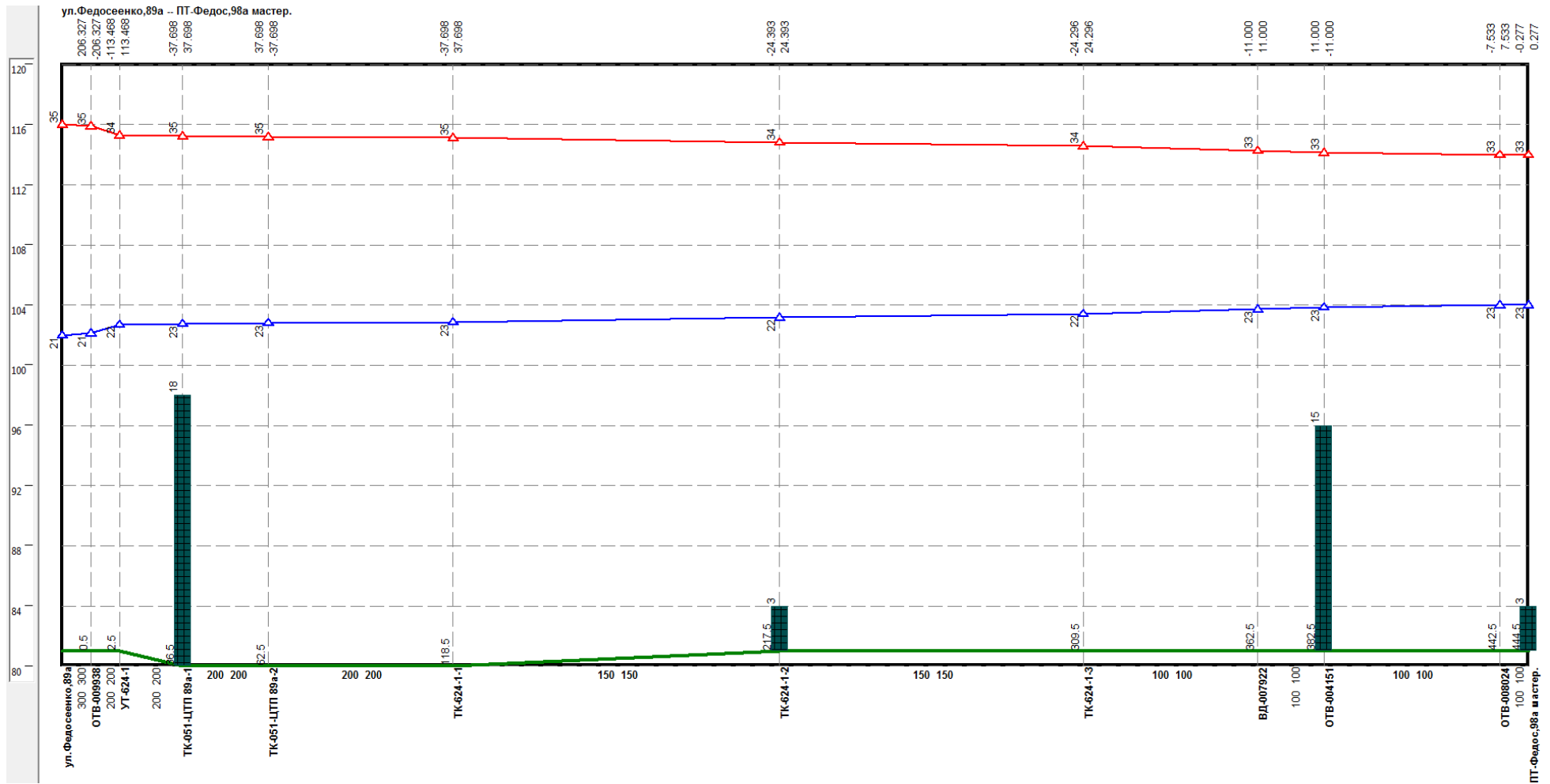
Рисунок 1.98 –Результат гидравлического расчета - график гидравлических режимов по пути теплоносителя от котельной ул. Федосеенко, 89-а до ПТ-Федос,98а мастер
