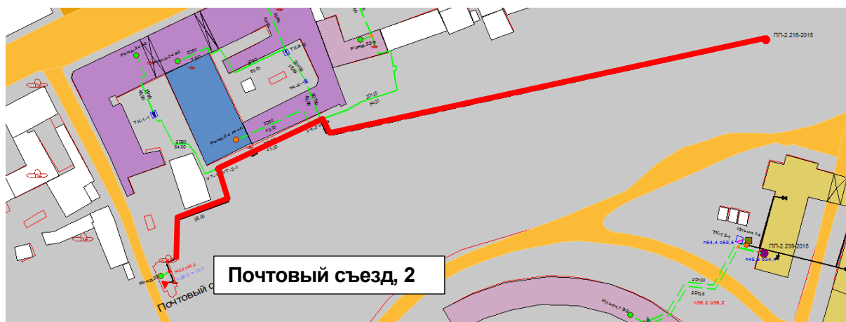
Рисунок 1.95 – Результат гидравлического расчета - расчетный путь теплоносителя от котельной Почтовый съезд, 2, 24 до ПТ-ПП-2.216-2015
