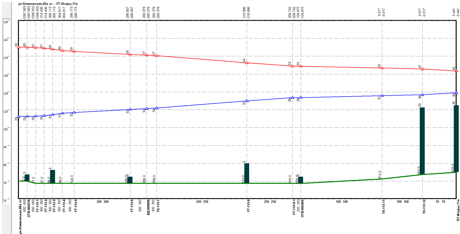
Рисунок 1.40 –Результат гидравлического расчета - график гидравлических режимов по пути теплоносителя от котельной Климовская, 86а до ПТ-Искры, 11а
