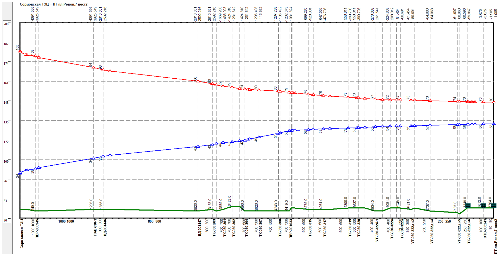
Рисунок 1.6 –Результат гидравлического расчета - график гидравлических режимов по пути теплоносителя от СТЭЦ до ПТ-пл.Револ,7 вест2
