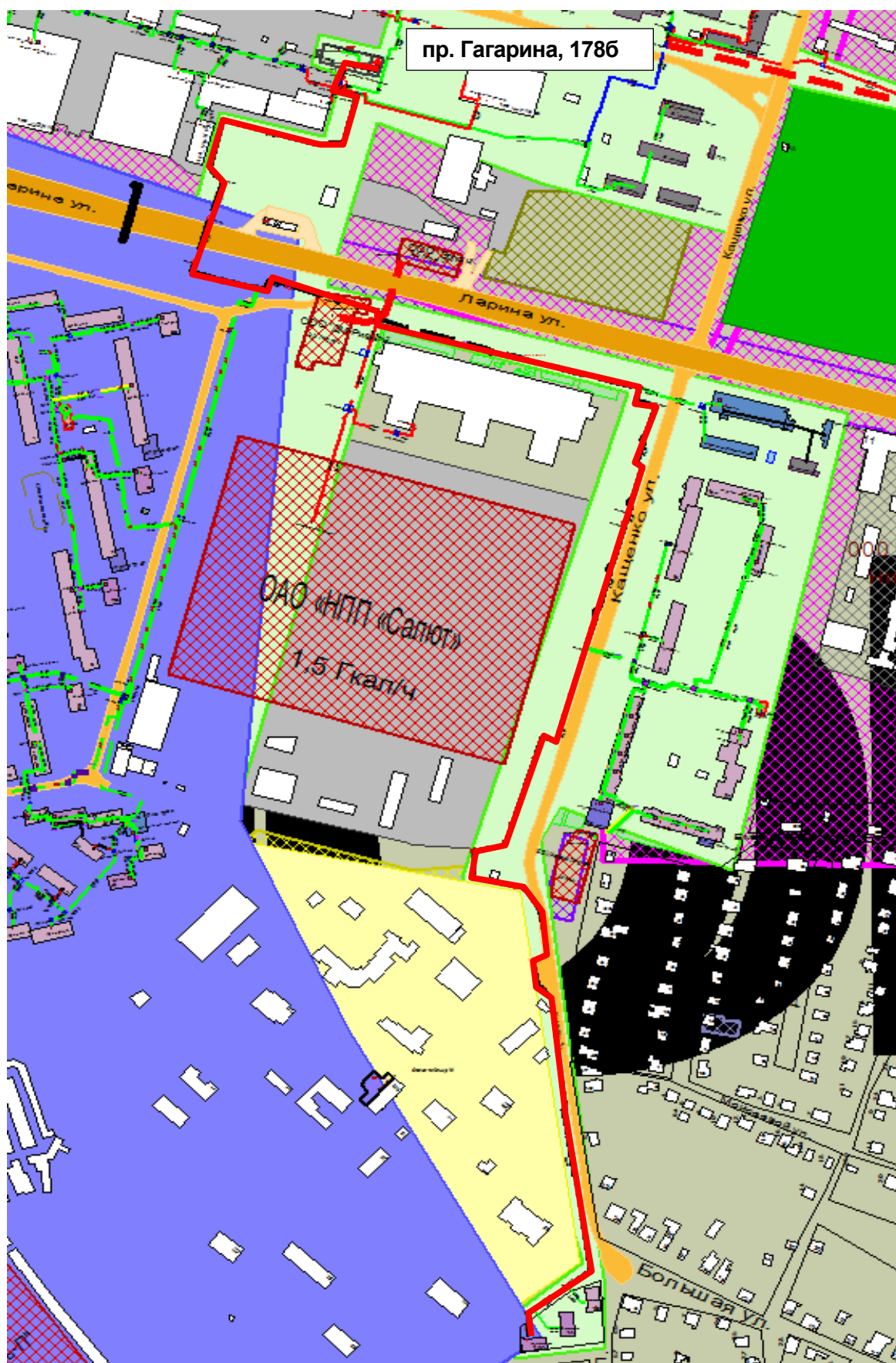
Рисунок 1.65 – Результат гидравлического расчета - расчетный путь теплоносителя от котельной пр. Гагарина, 1786 до ПТ-Кащенко,14а
